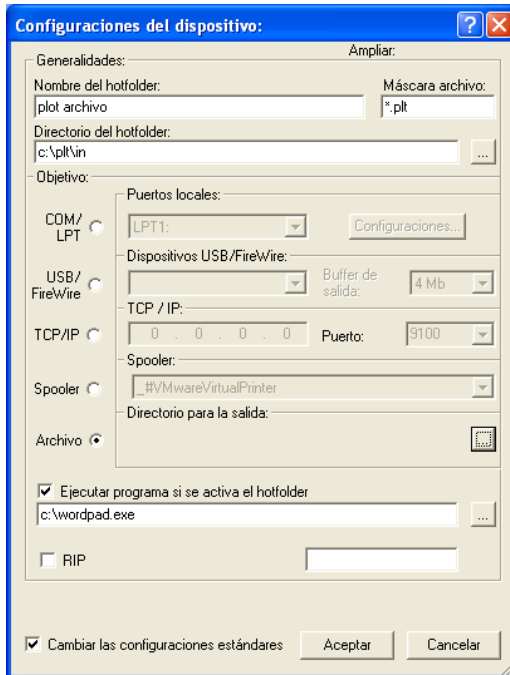
Fig. 7.2-3: Ejemplo para configuraciones de dispositivos de un Hotfolder
