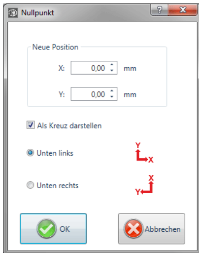
Abb. 4.5-12: Der Nullpunkt-Dialog
