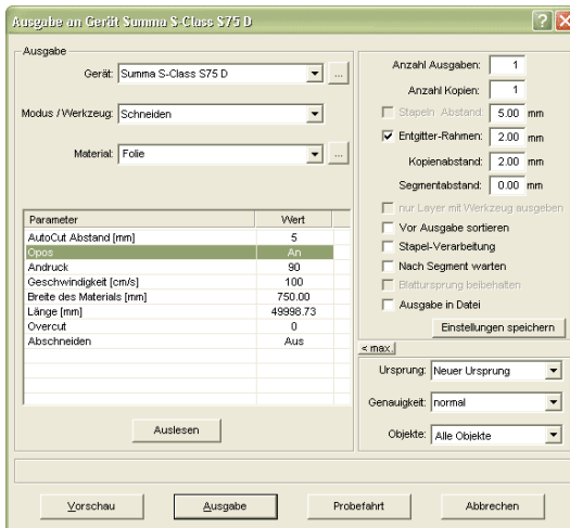
Abb. 4.10-5: Parameter-Einstellung "Opos=AN" bei am Beispiel Schneideplotter Summa S-Class
